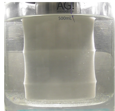
図1 回転する円管の表面に析出した脂肪酸の層状結晶
